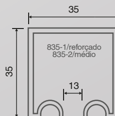
35x35 côncavo TRP-835
