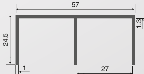
Perfil superior para guia TPM - 807-1
