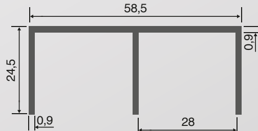
Perfil superior leve para guia TPM - 807-2
