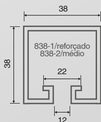
38x38 reto TRP-838
