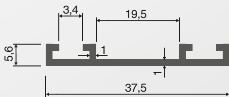
Perfil inferior para roupeiro TPM - 805-2
