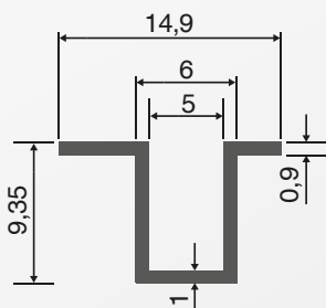
Perfil inferior para roupeiro TPM - 805-2
