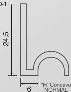
35x35 côncavo TRP-835
